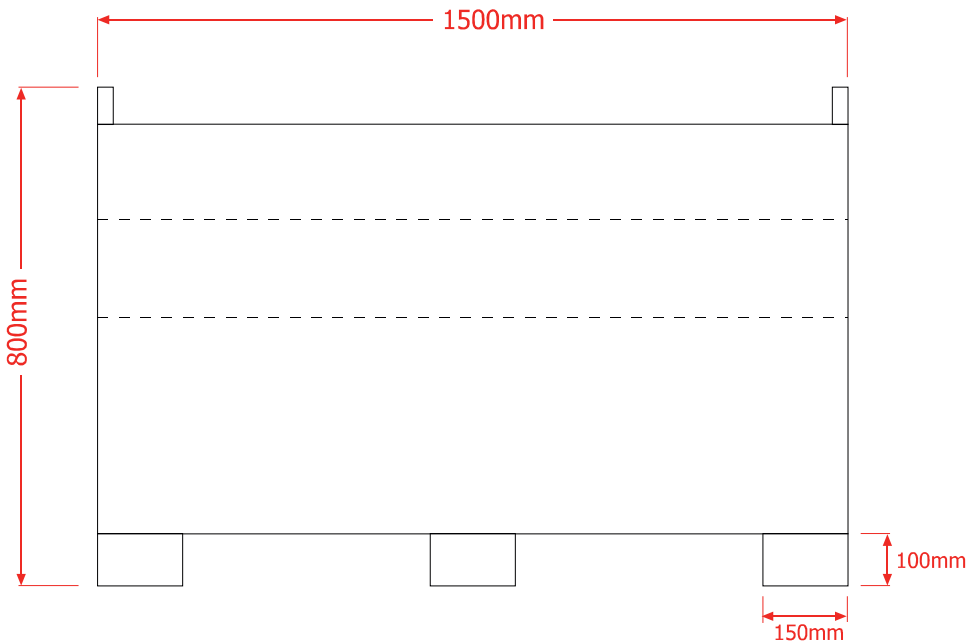
منظر أمامي
